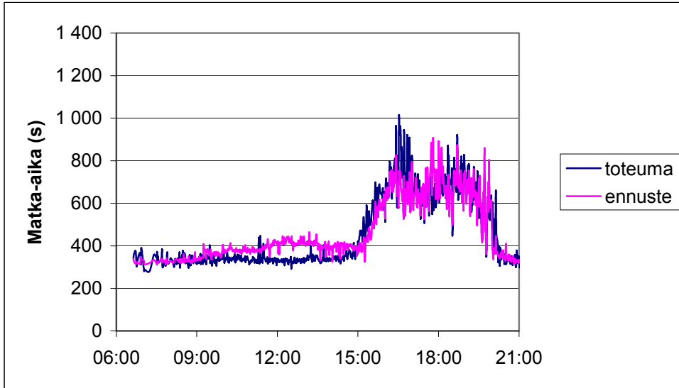
Kuva 14. Kaikkien perjantaipäivien toteumien ja ennusteiden keskiarvot Seesta–Vierumäki-tiejakson 15 minuutin ennustemallilla testausaineistossa.
