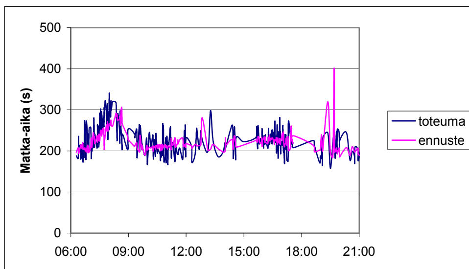
Kuva 13. Toteumat ja ennusteet Perkkää–Otaniemi-tiejakson 15 minuutin ennustemallilla testausaineistossa maanantaina 13.9.2004.
