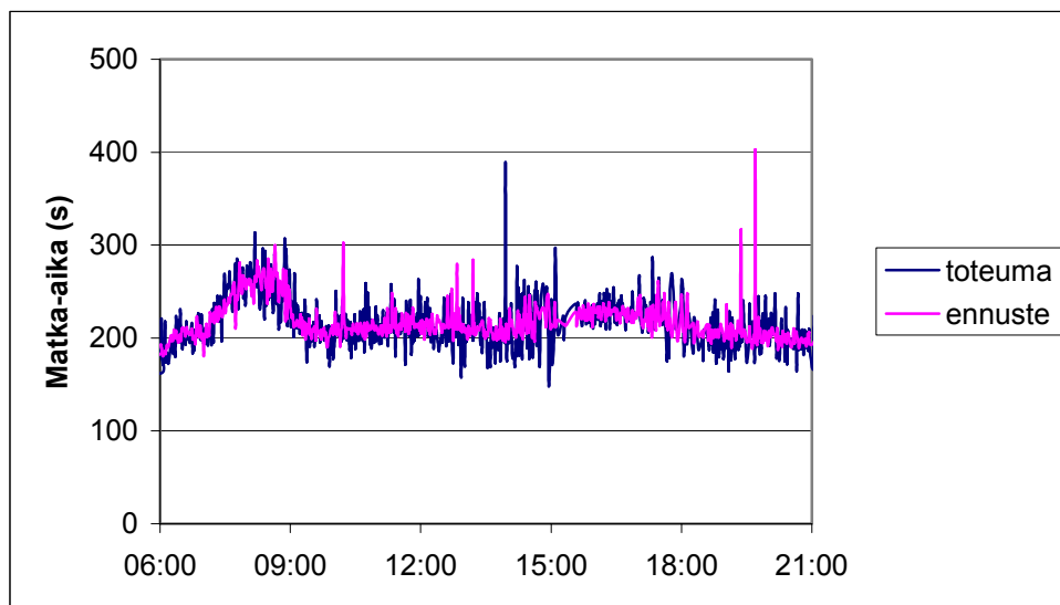
Kuva 12. Kaikkien maanantaipäivien toteumien ja ennusteiden keskiarvot Perkkää–Otaniemi-tiejakson 15 minuutin ennustemallilla testausaineistossa.
