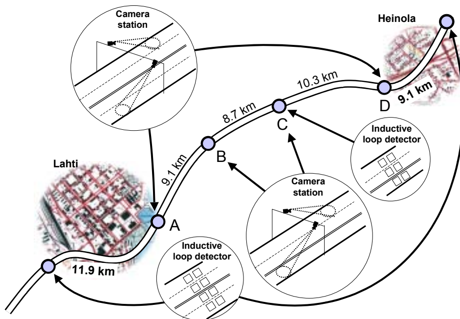
Kuva 5. Kaistojen lukumäärät, tieosien pituudet ja liikenteen seurantalaitteet valtatie 4 tutkimuskohteessa. Kamerapisteet olivat Kymijärvellä (A), Seestassa (B), Vierumäellä (C) ja Heinolassa (D).
